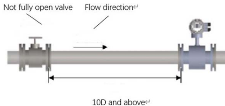
Fig.7 전자기 유량계 앞부분에 완전히 개방되지 않은 밸브가 설치되어 있을 경우
