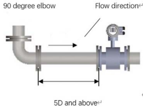
Fig.6 유량계 전면에 90° 엘보 직선관 부분이 있는 경우
