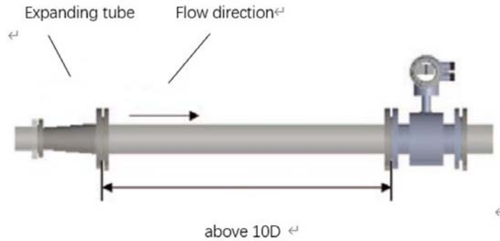
Fig.8 유량계 전면에 확경관이 설치되어 있는 경우
