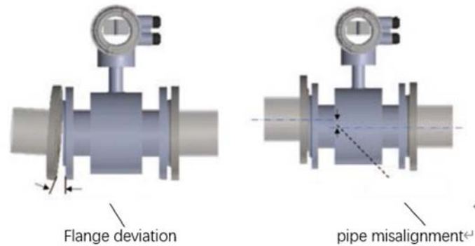
Fig. 3 유량계 배관
