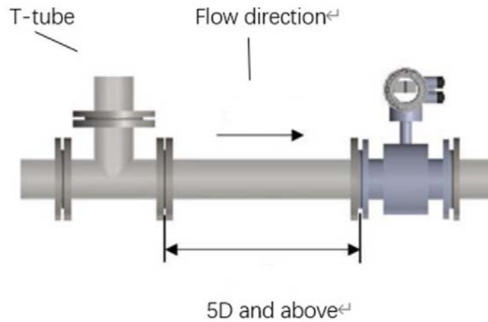
Fig.5 유량계 전면에 T-pipe 직선관 부분이 있는 경우
