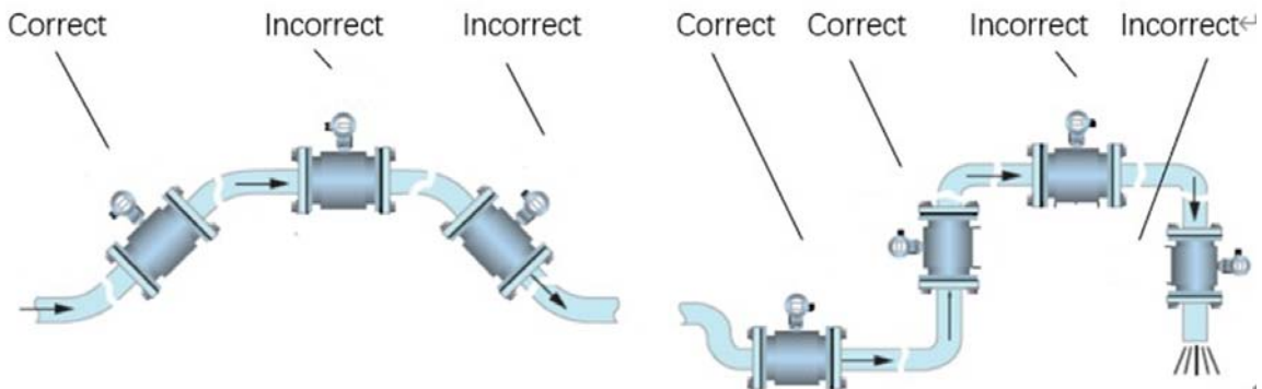
Fig.1 설치 위치
