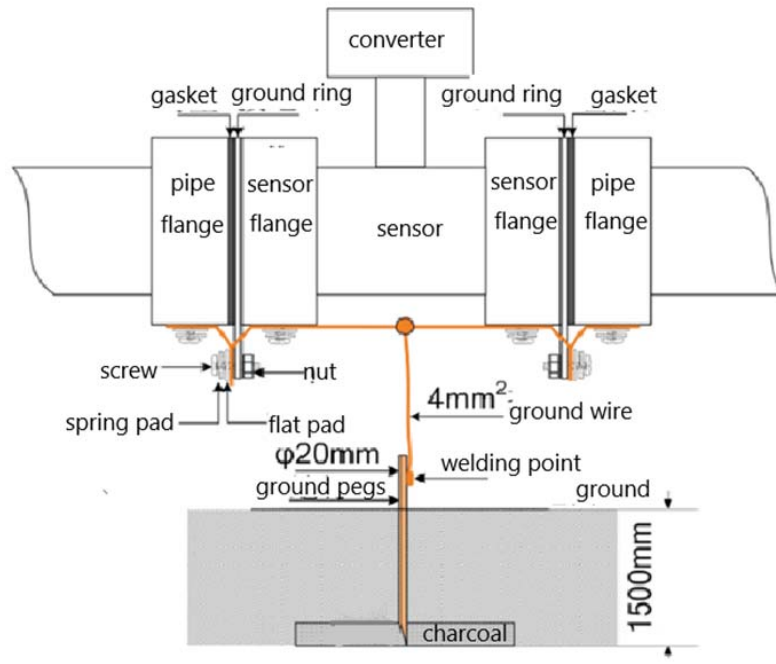
Figure 9 컨버터 접지 설명도
